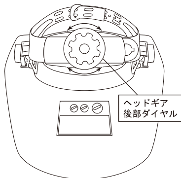
図2. 締め付けの調整
